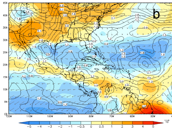
MSLP (hPa)
