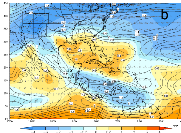
MSLP (hPa)
