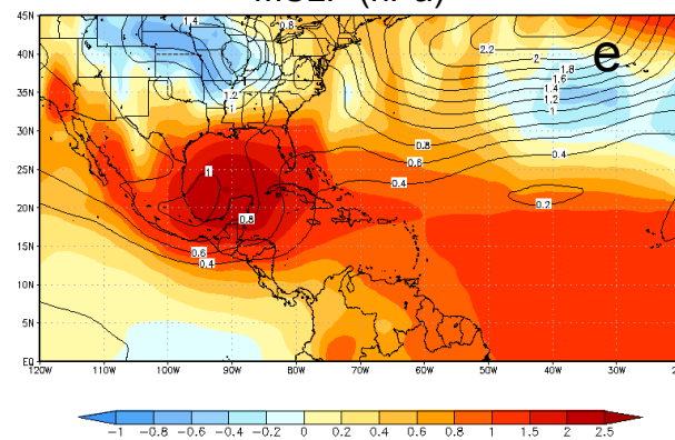
MSLP (hPa)
