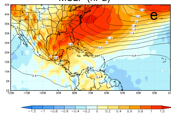
MSLP (hPa)
